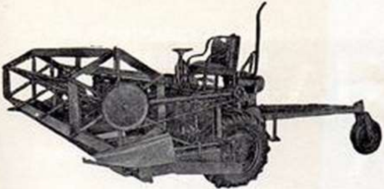
PLATAFORMA HILERADORA "CMC" Aplicada al chasis tractor, 16 pies de corte. Descarga al centro mediante dos lonas de tela engomada. Su patín de acero permite trabajar casi a ras del suelo.
