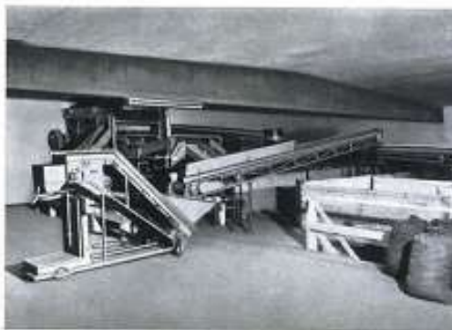
Stat. vollautomatische Kartoffelboxen- beschickungsanlage mit Sortierung.
