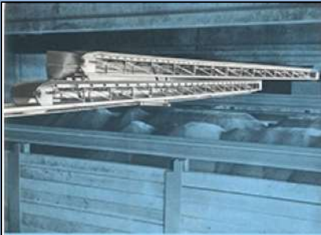
Förderanlage für Dünger schwenkbar und verschiebbar.
