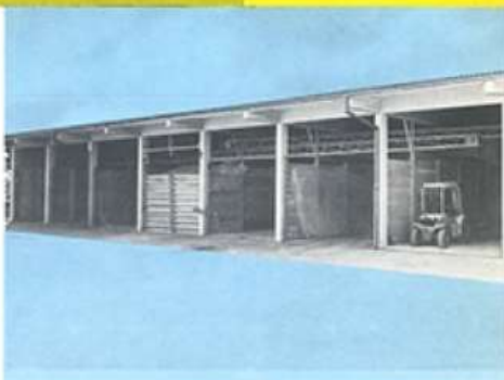
Ansicht einer Düngelagerhalle mit einer GAMO-Beschickungsanlage.
