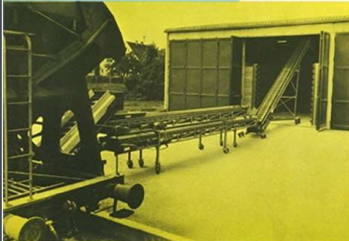
Mit der GAMO-Schwenk- und Verschiebeanlage können alle Boxen gleichmäßig beschickt werden. Die Schwenkung geschieht mittels Seilwinden vom Boden aus.
