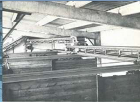
Mit der GAMO-Schwenk- und Verschiebeanlage können alle Boxen gleichmäßig beschickt werden. Die Schwenkung geschieht mittels Seilwinden vom Boden aus.
