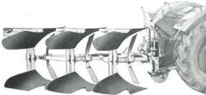
ADDD-A mit KS-Panzerstahl-Streichblechen
