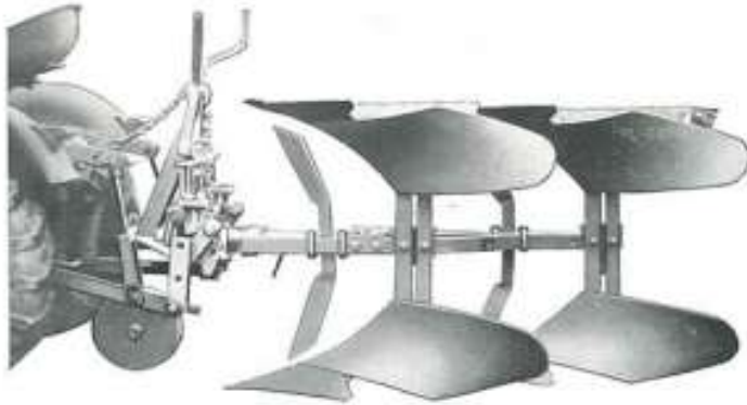
AZDD-A mit KS Panzerstahl-Streichblechen
